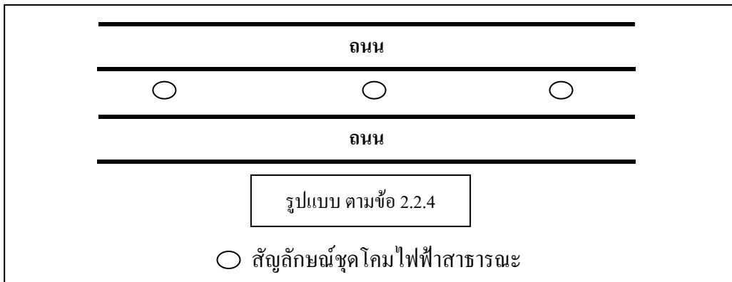
รูปที่ 2-1 การกำหนดรูปแบบ และจุดติดตั้งไฟฟ้าสาธารณะตามแนวถนนตามข้อ 2.2
